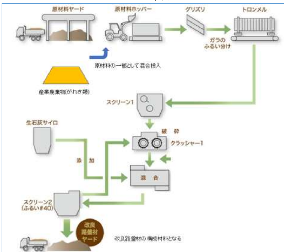
処理工程図
